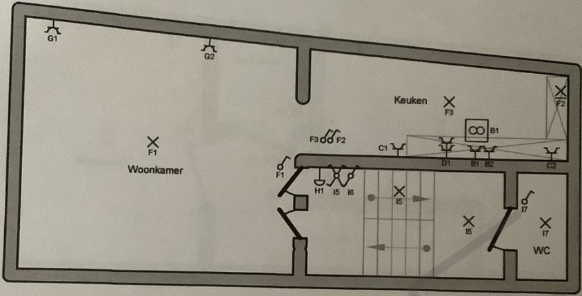
1e Verdieping
