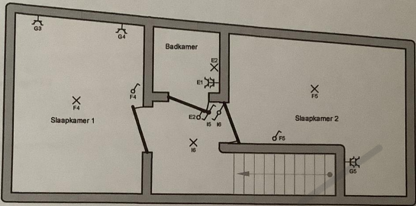
2de Verdieping
