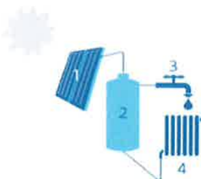
1. Zonnecollector | 2. Opslagvat warm water | 3. Sanitair warm water | 4. Afgifte-element voor ruimteverwarming (optioneel)
