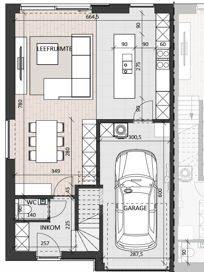
GELIJKVLOERS
