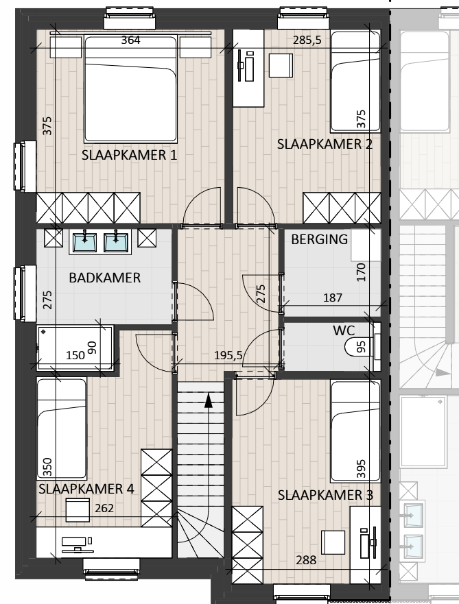
1e VERDIEPING
