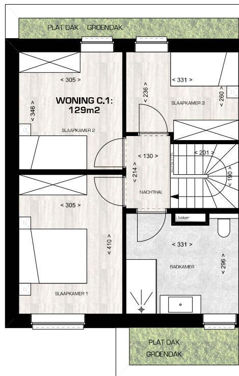
VERDIEPING
