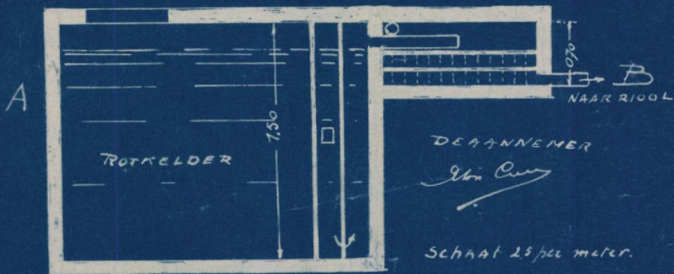
DOORSNEDE A-B
