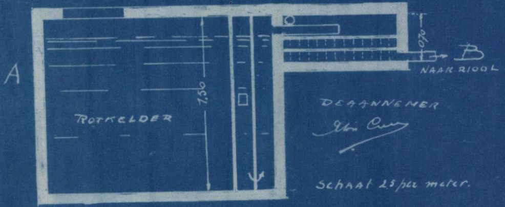
DOORSNEDE A-B
