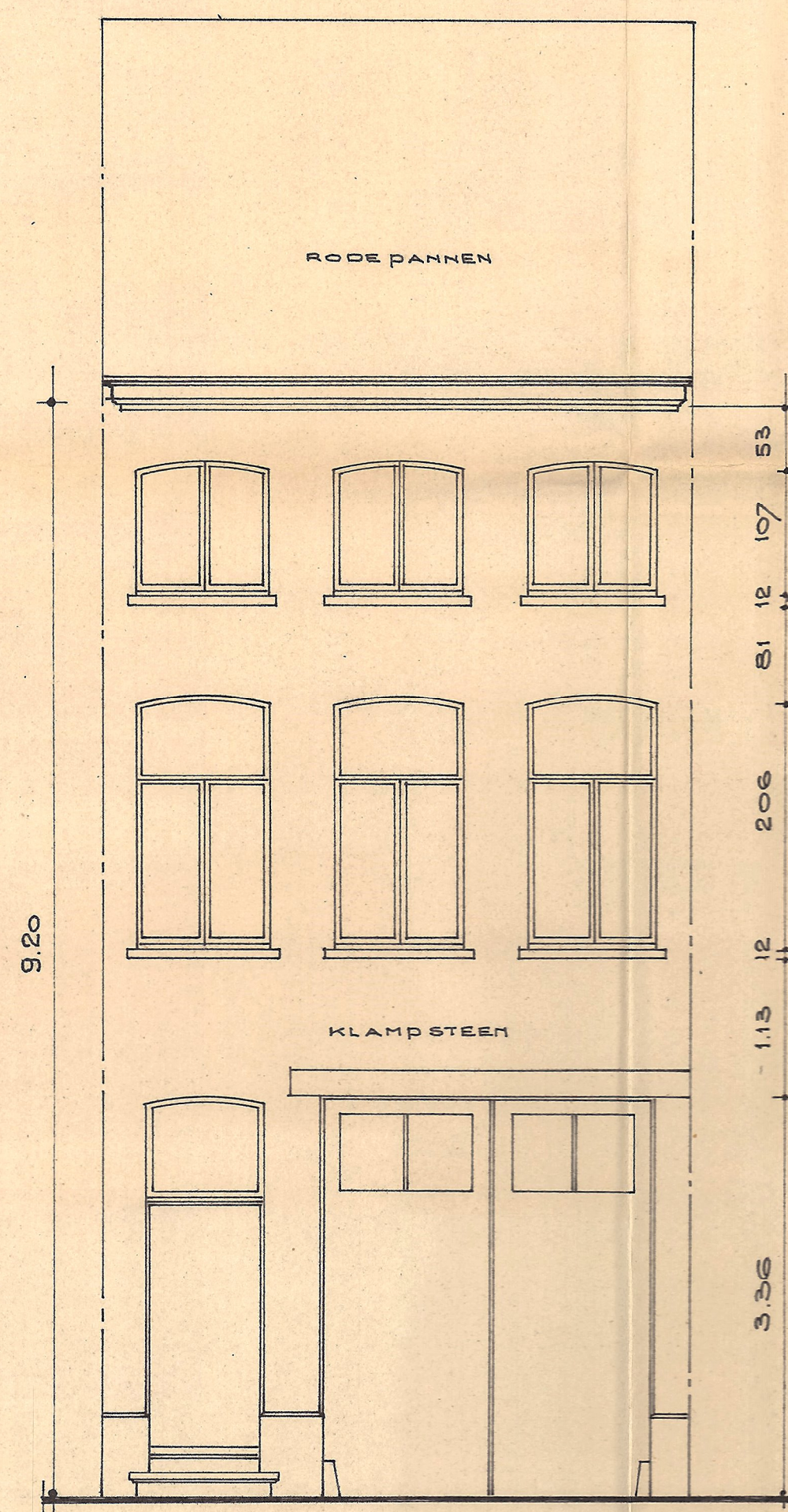
BESTAANDE GEVEL
