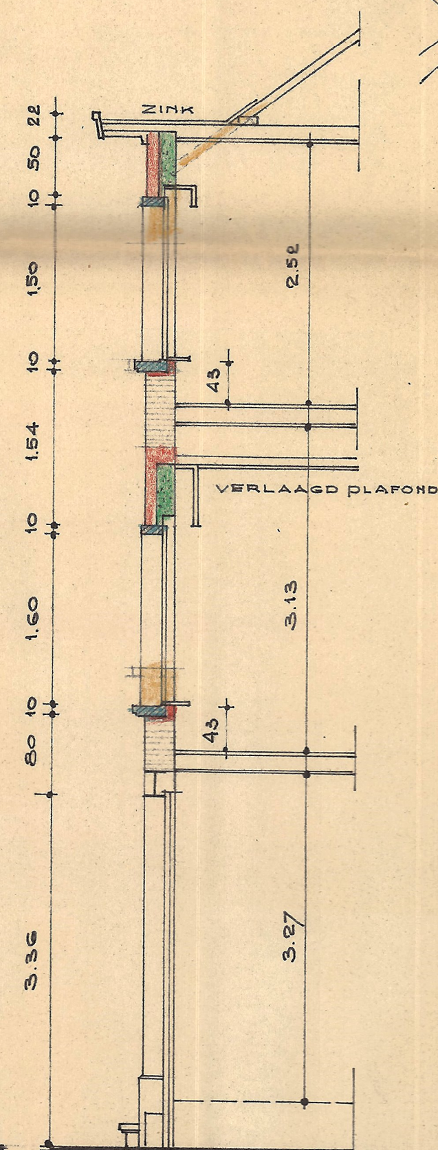
DOORSNEDE
