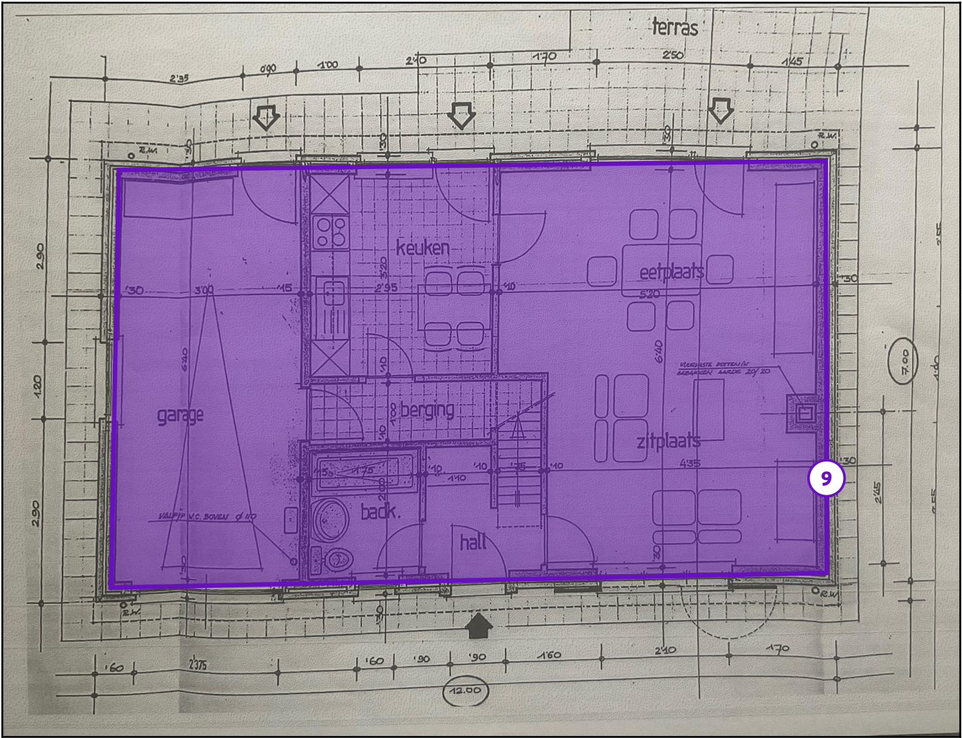
Legende van plan 1.2: Gelijkvloers : plafonds
