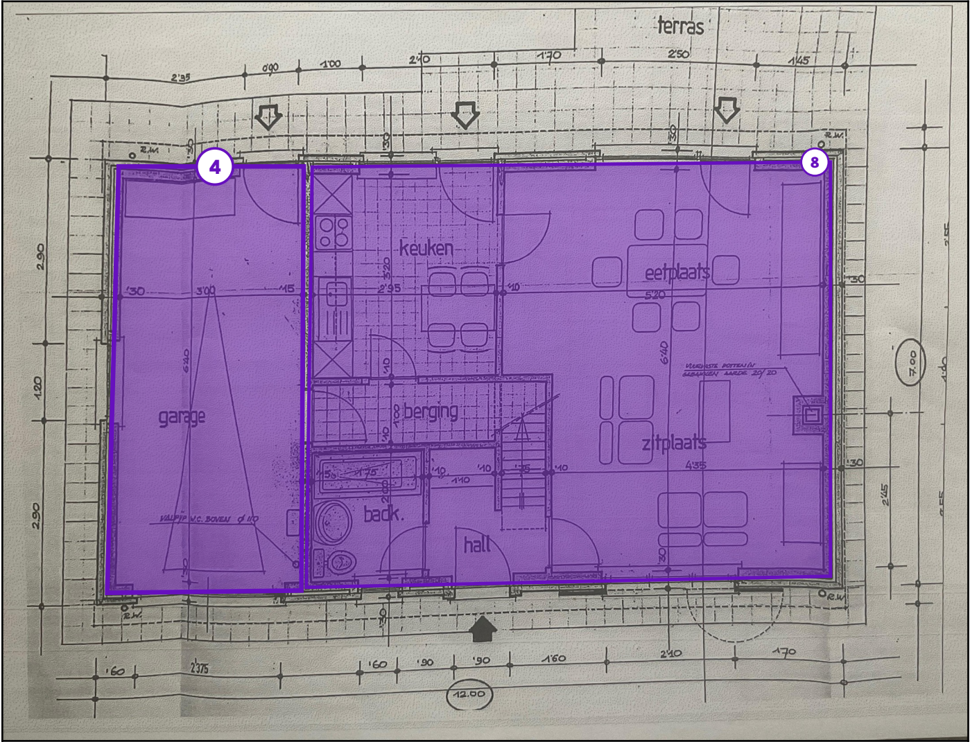
Legende van plan 1.3: Gelijkvloers : vloeren
