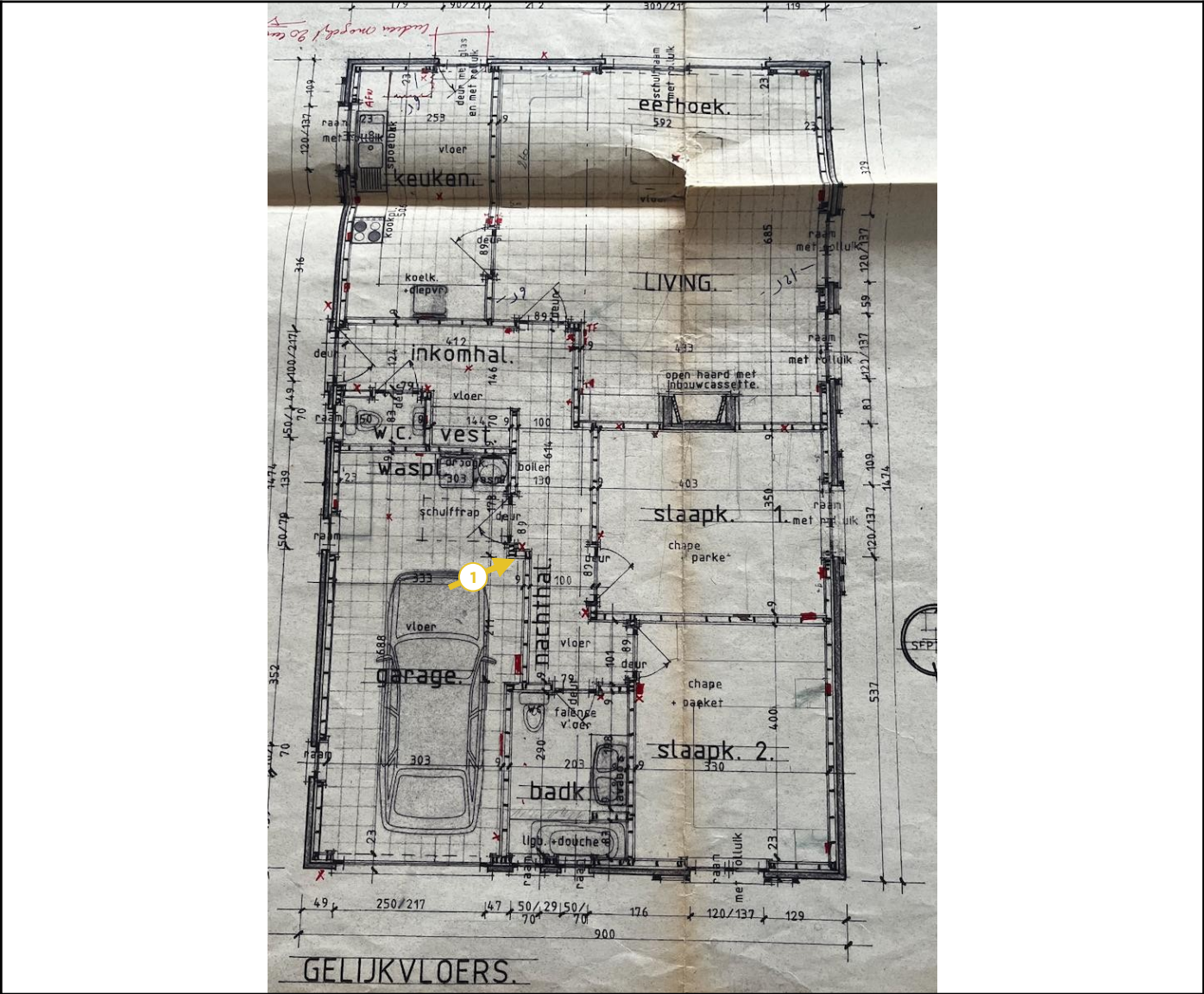
Legende van plan 1.1: Bakeliet zekeringskast
